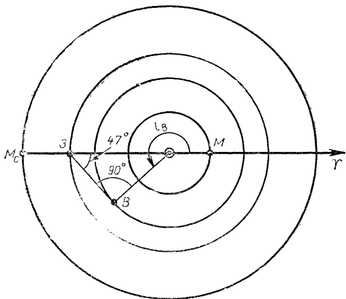
Рис. 6. Конфигурации планет
