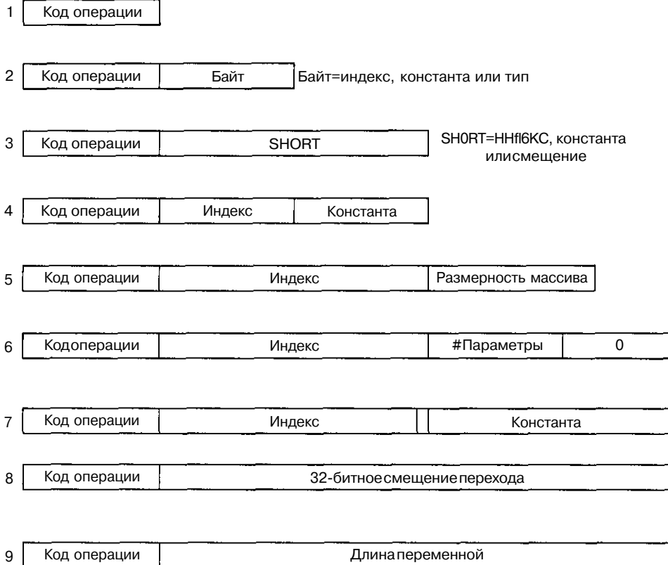
Рис. 5.11. Форматы команд JVM
