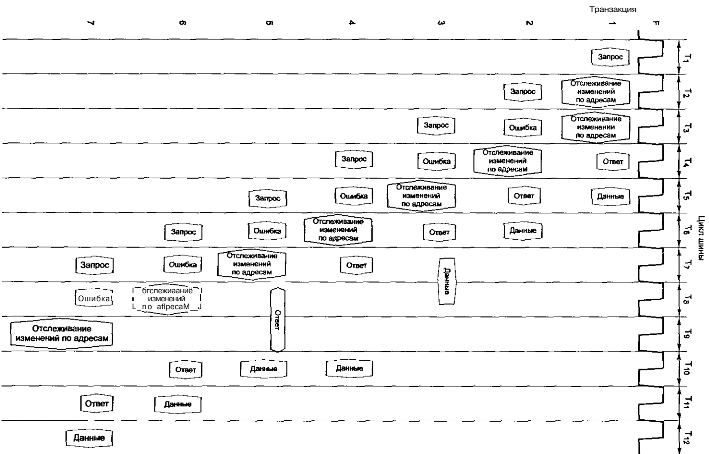
Рис. 3. М. К О в е р н ы й р е ж и м ш и н н ы п а м я т и в д и с т а н ц и о н н о м с о о б щ е н и и
