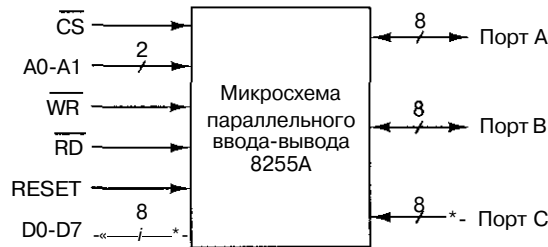
Рис. 3.51. Микросхема 8255А
